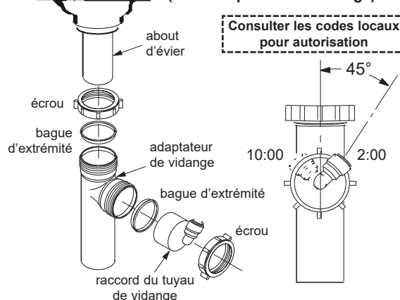
B – RACCORDEMENT DES EAUX USÉES (avec adaptateur de vidange)
