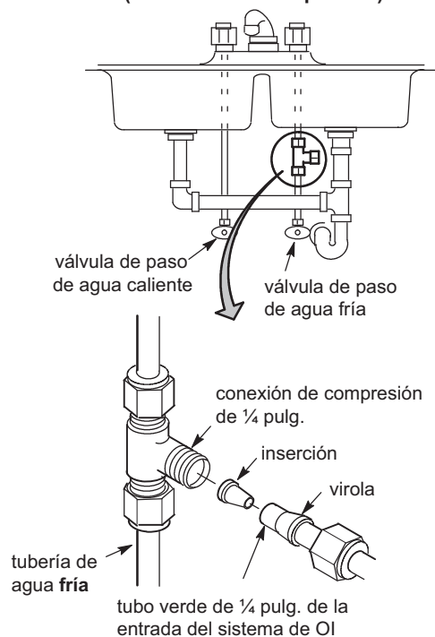
FIGURA 1 CONEXIÓN TÍPICA DEL SUMINISTRO DE AGUA (con unión de compresión)
