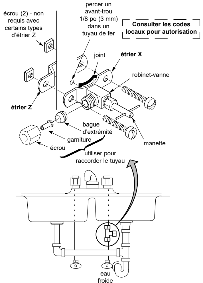
FIGURE 9 - RACCORDEMENT DE L'ALIMENTATION D'EAU (avec robinet-vanne à étrier)
